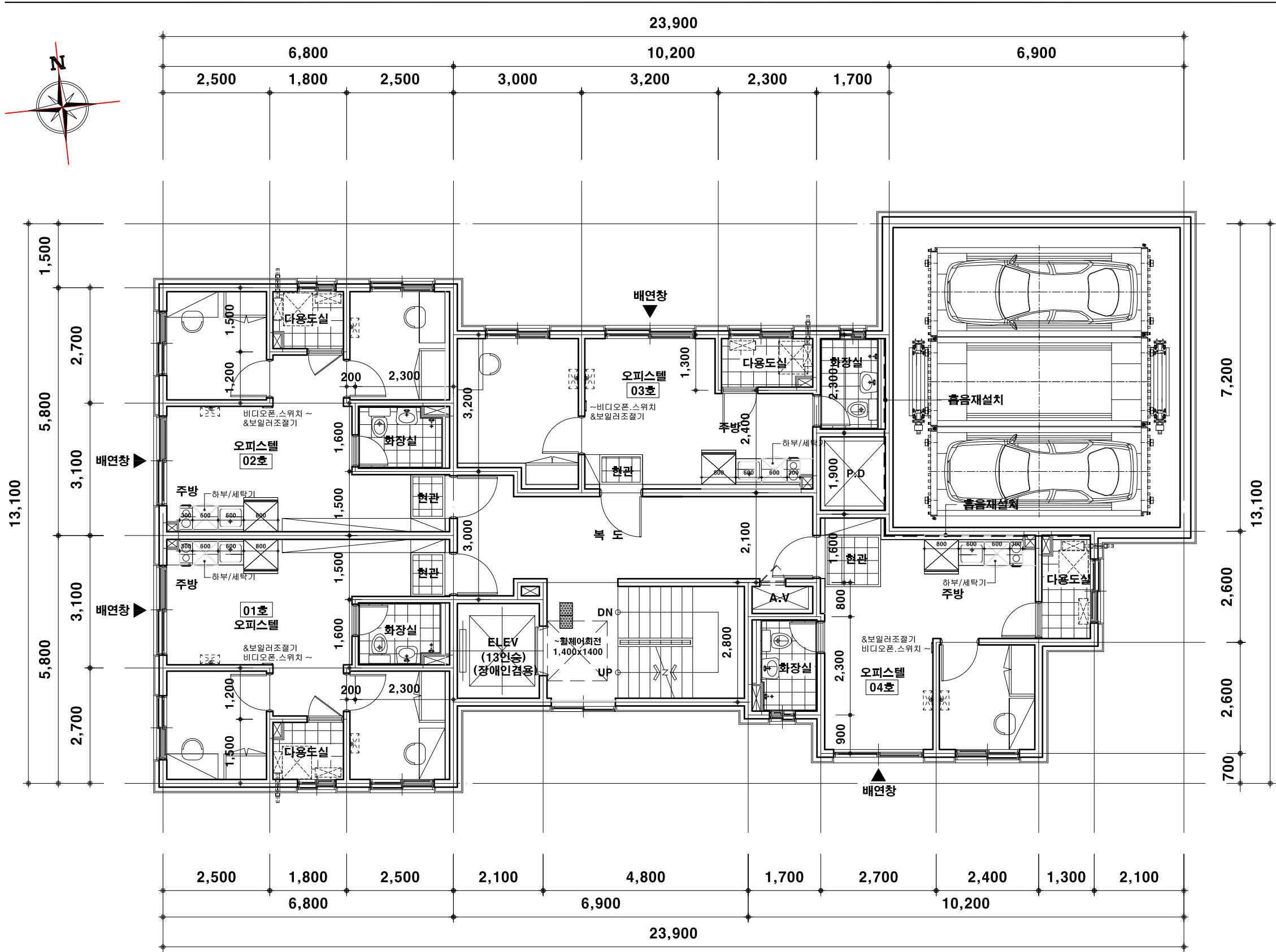
2~10층 평면도 SCALE : 1/100
