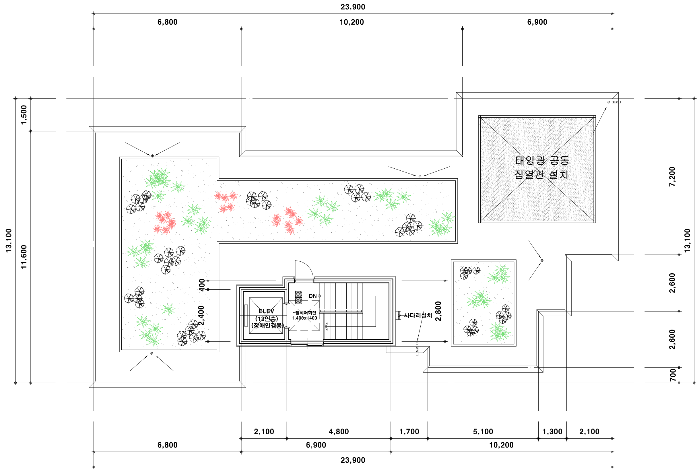
지붕 평면도 SCALE : 1/100
